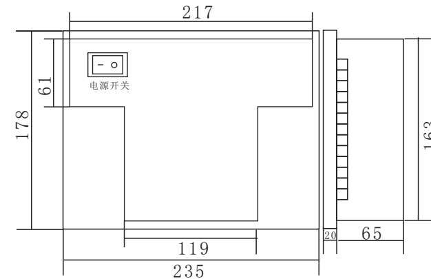
外形尺寸: 235×178×85
